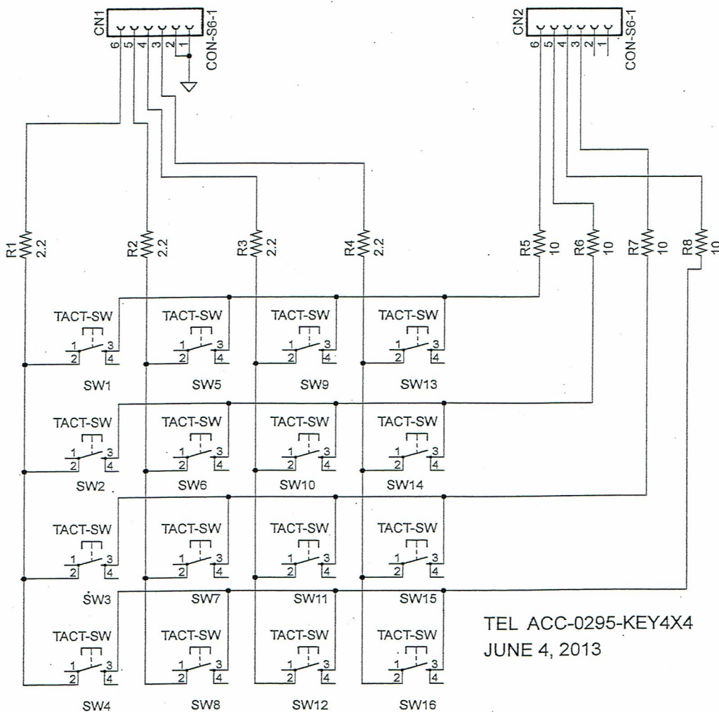
キーパッド(品番ACC-0295-KEY4X4)回路図
